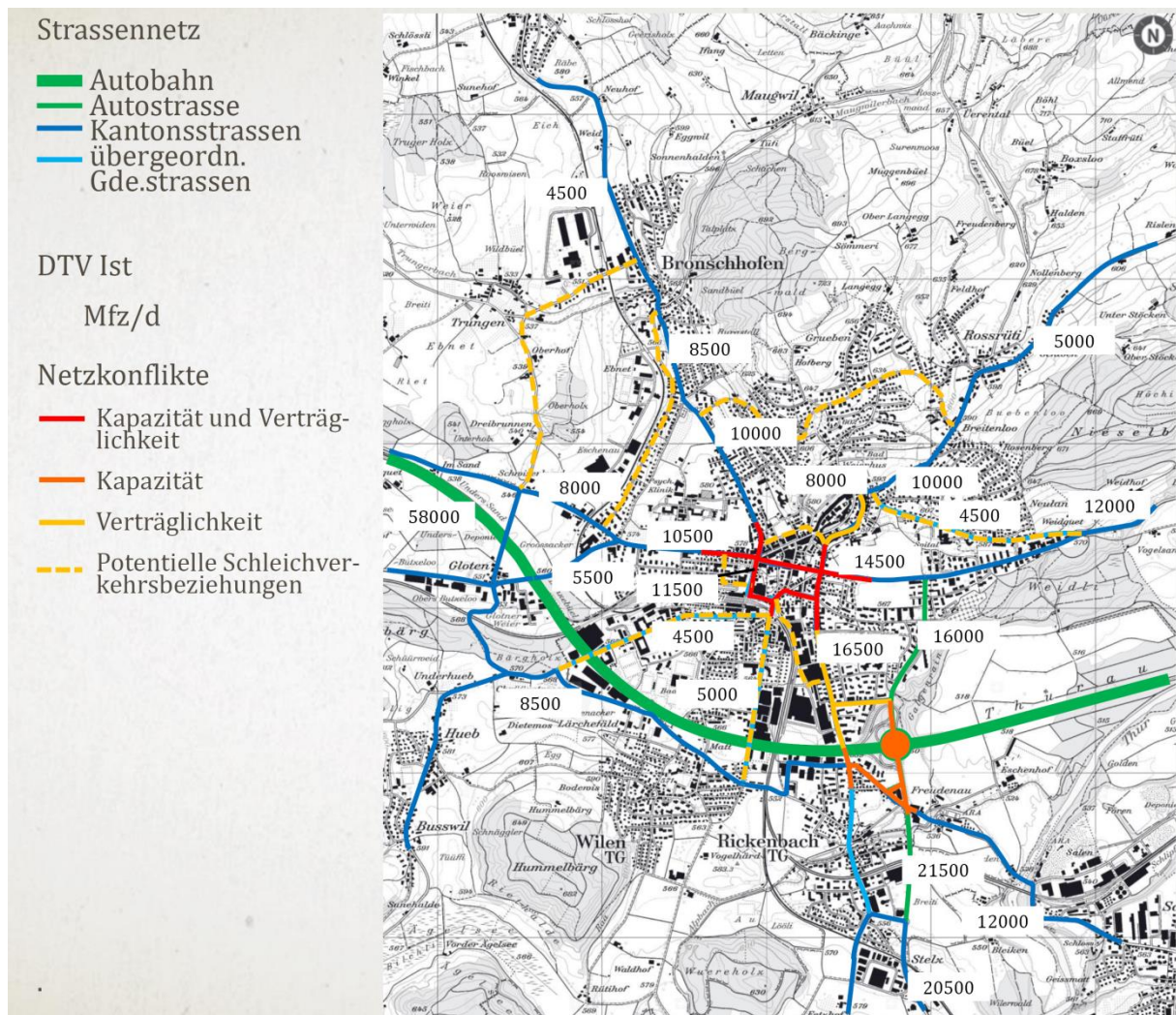
Abbildung 10: Übersicht Probleme auf dem Strassennetz
